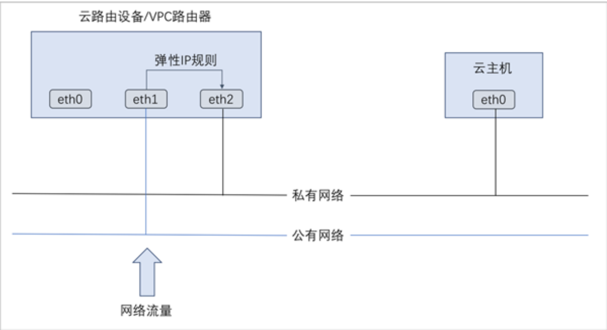
图 378: 云路由网络/VPC下弹性IP的应用场景
