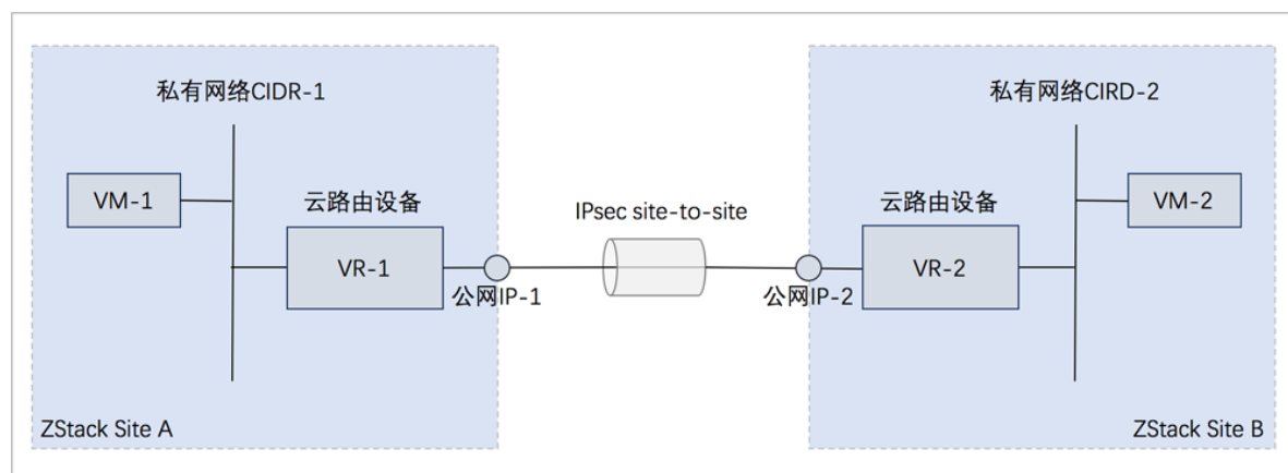
图 354: 云路由网络下IPsec隧道应用场景
