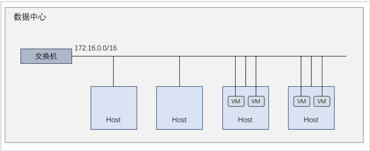
图 365: 二层扁平网络
