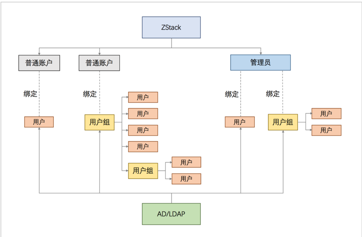
图 723: ZStack-AD/LDAP绑定关系
