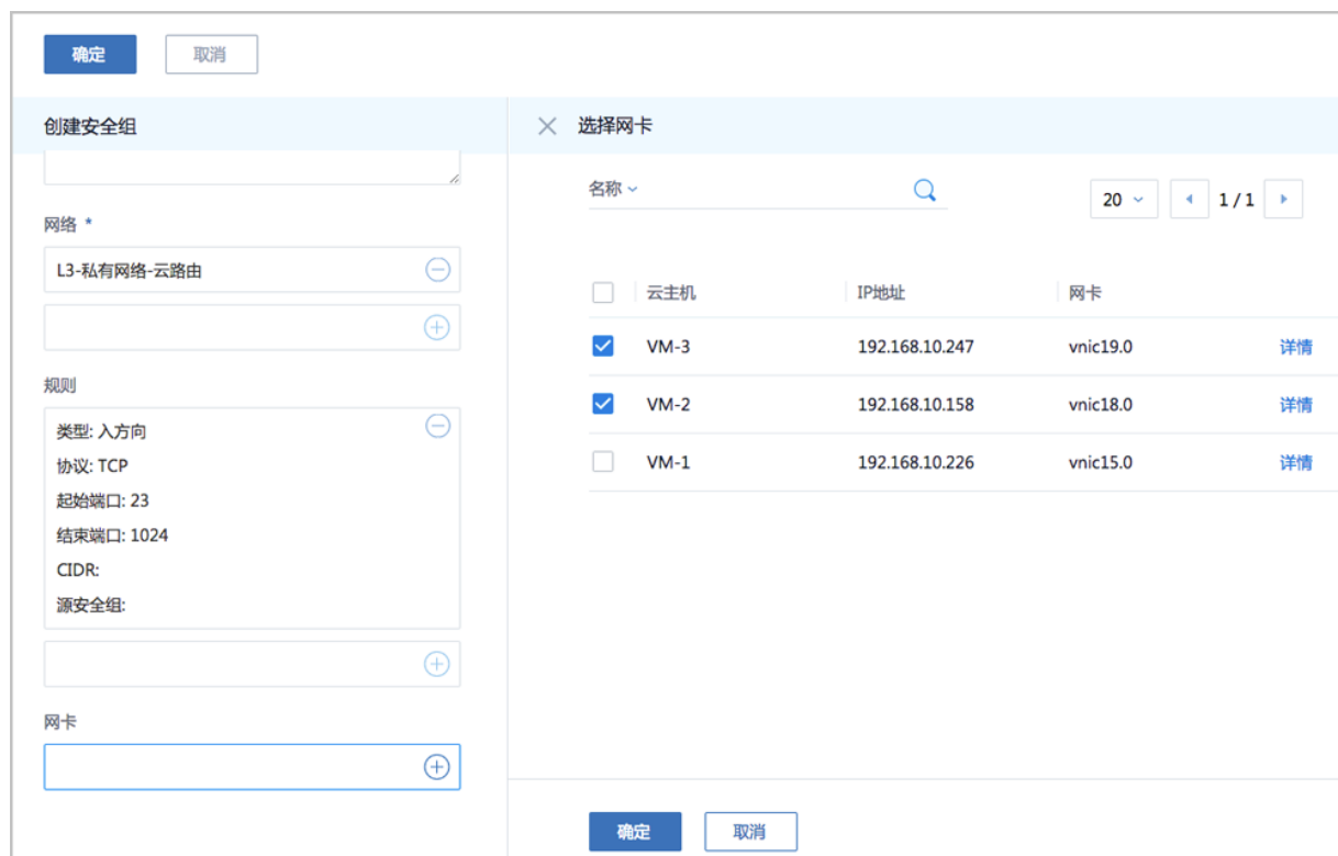
图 329: 添加云主机网卡到安全组
