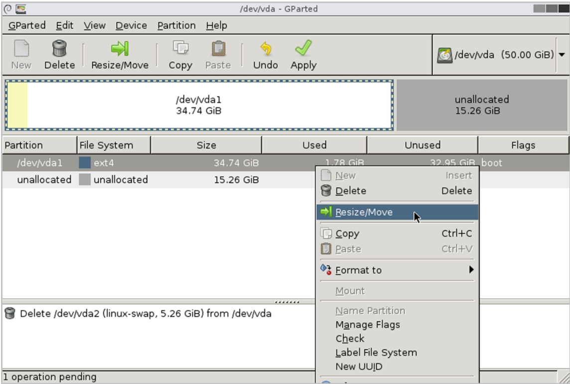
图 131: 扩展ext4从35G至46G
