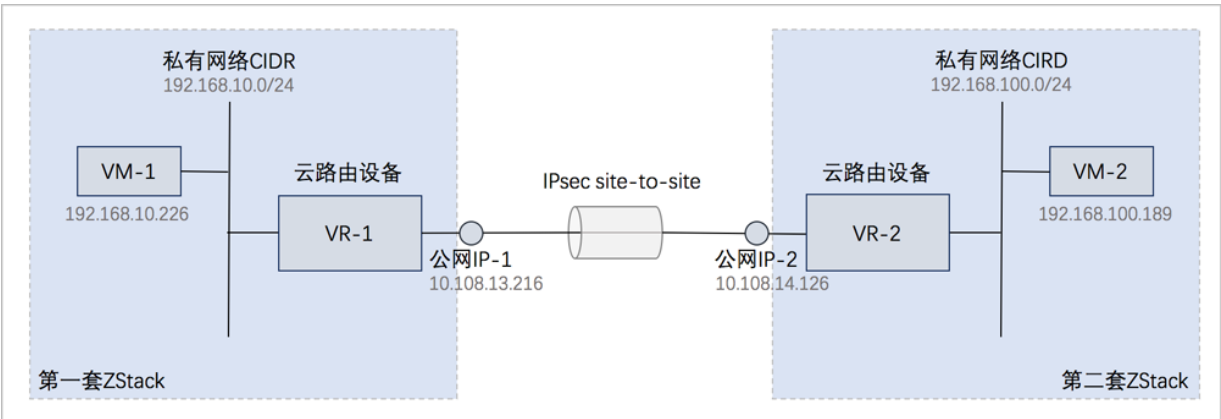
图 503: IPsec隧道网络架构图
