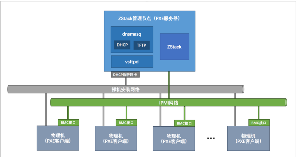
图 237: 裸机安装网络(见灰色) 规划示意图
