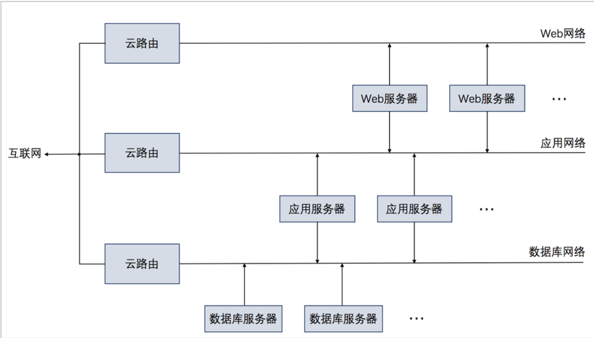
图 419: 多层Web服务器网络架构图
