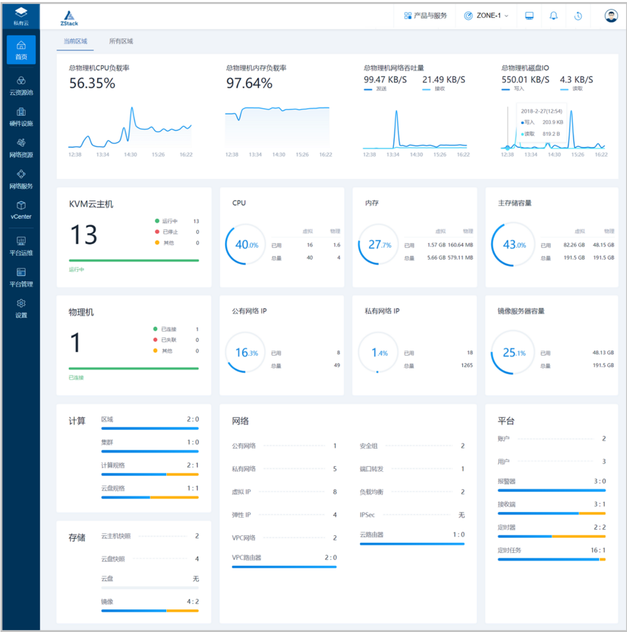
图 90: 首页
