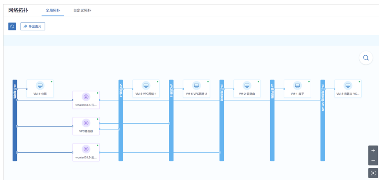
图 296: 全局拓扑
