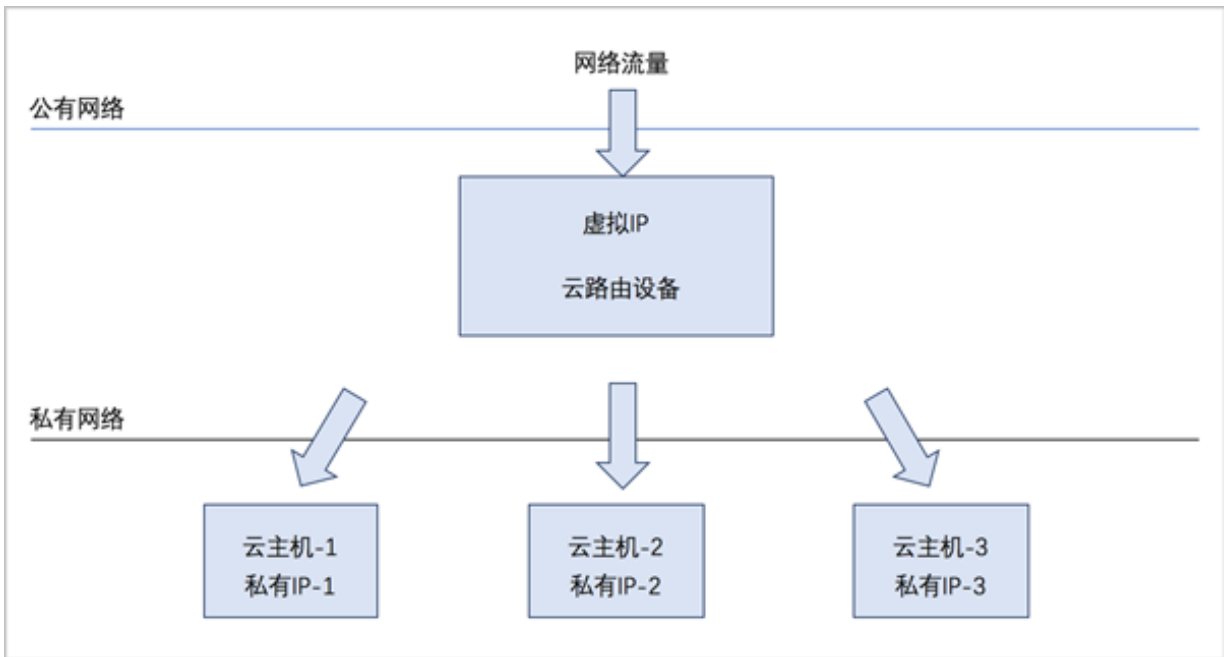
图 491: 虚拟IP-负载均衡
